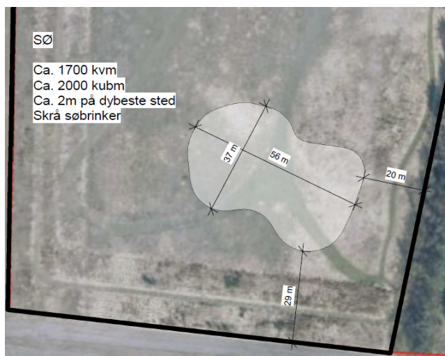
Figur 2. Ansøgers projekttegning over vandhullet.
